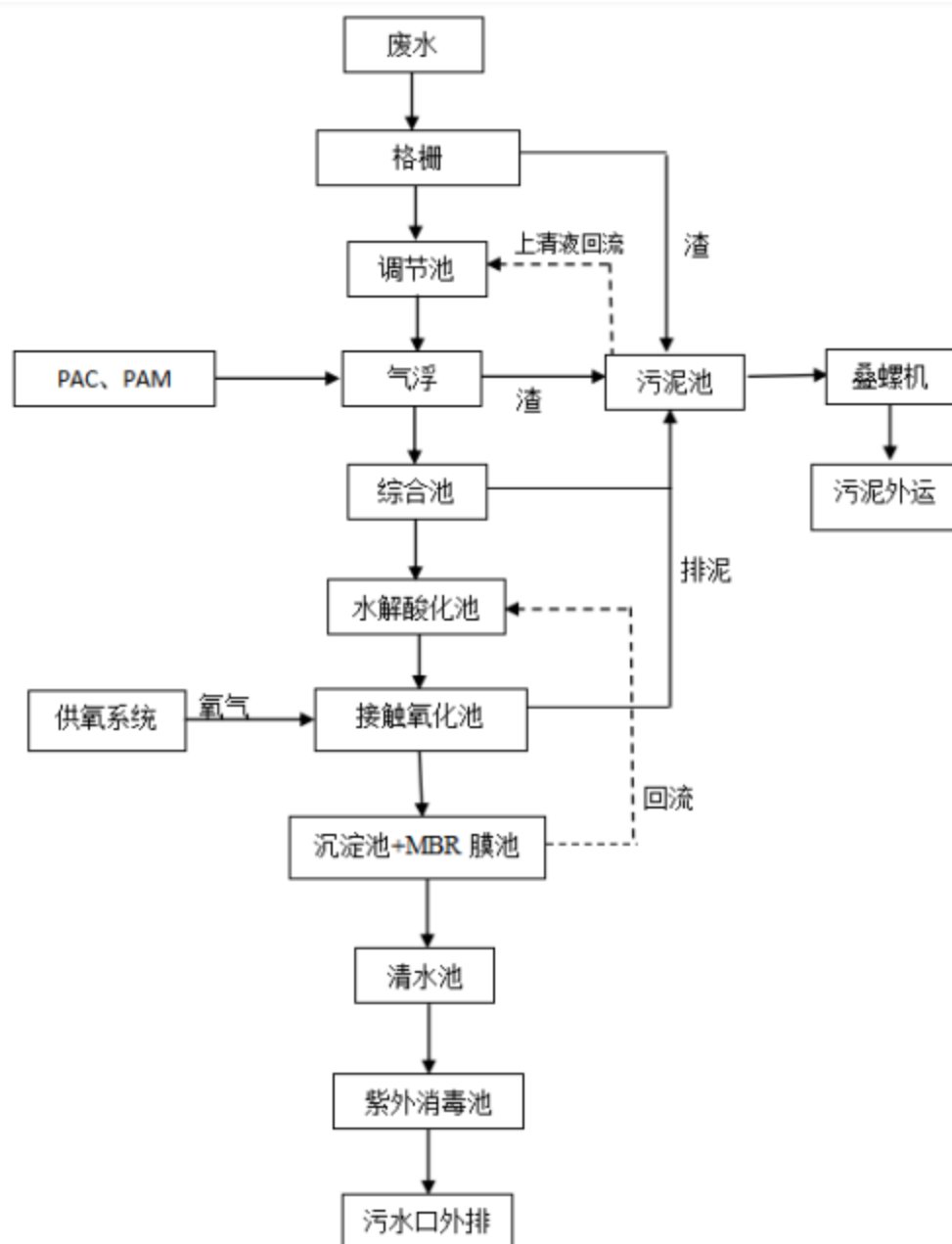
图 6.1-1 污水处理站处理工艺流程图
