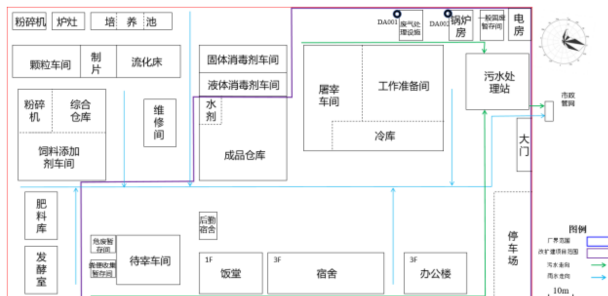
图 3.2-3 改扩建项目雨污水走向图
