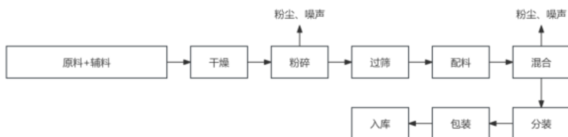
图 3.1-8 饲料添加剂工艺流程图
