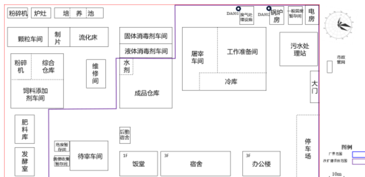
图 3.2-2 改扩建项目平面布置图
