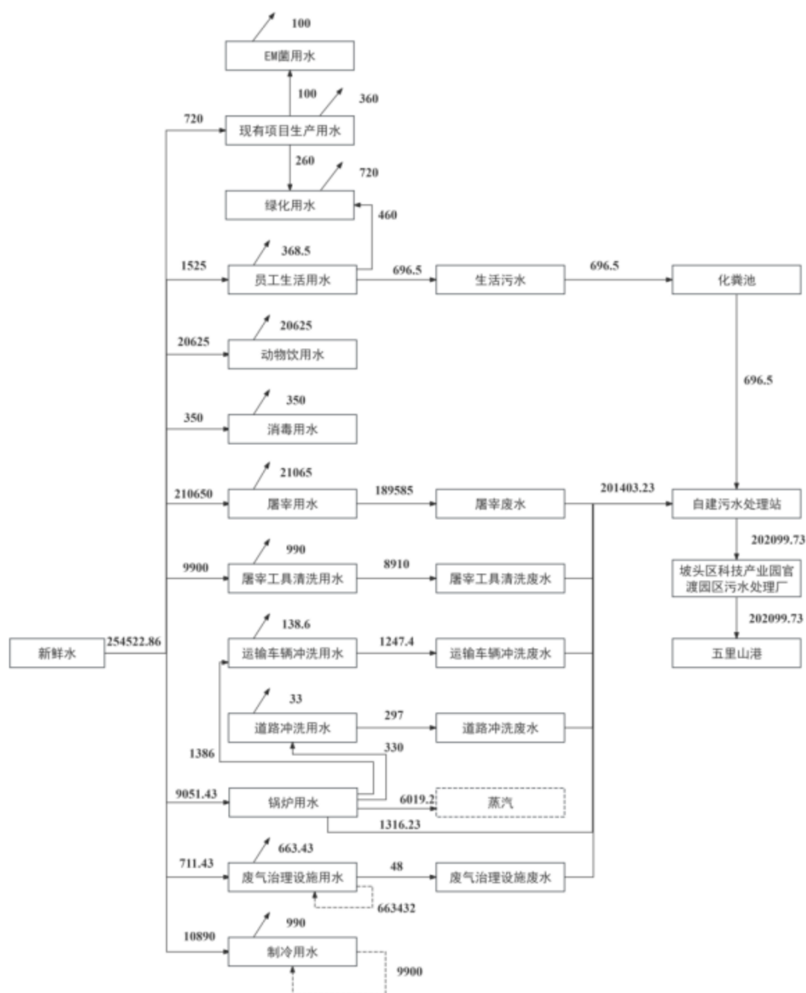
图 3.2-3 改扩建后全厂水平衡图 (单位: \text{m}^3/\text{a} )
