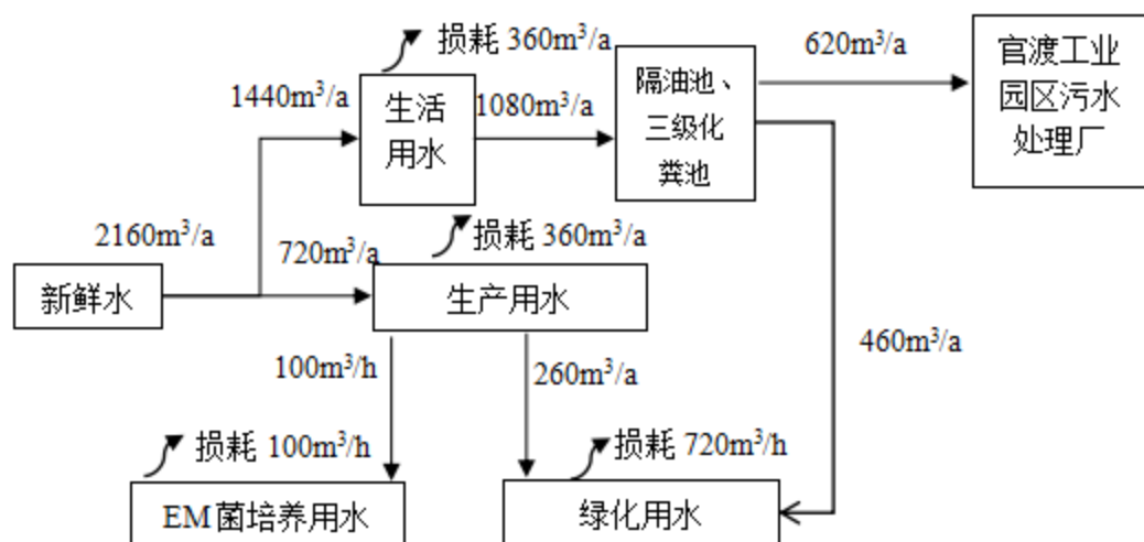
图 3.1-2 现有项目水平衡图 (m³/a)
