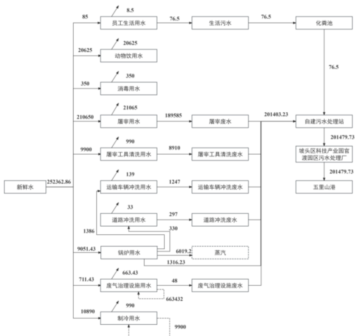
图 3.2-2 改扩建项目水平衡图 (单位: \text{m}^3/\text{a} )
