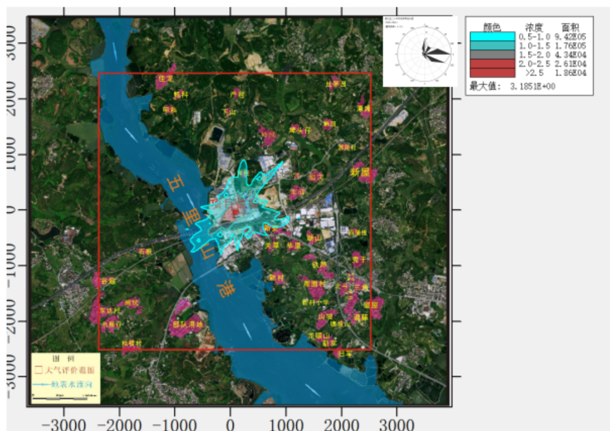
图 5.2-32 非正常工况下硫化氢小时均值贡献值预测图 (单位: \mu\text{g}/\text{m}^3 )
