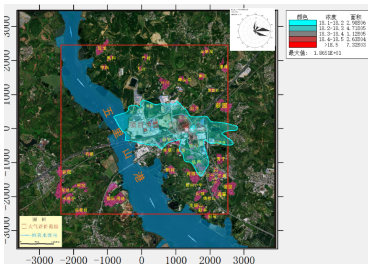
图 5.2-22 正常工况下二氧化硫日均值叠加背景值预测图 (单位: \mu\text{g}/\text{m}^3 )
