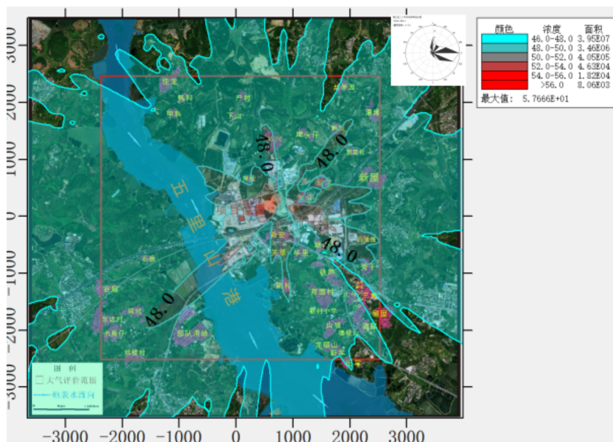
图 5.2-26 正常工况下 M_{2.5} 日均值叠加背景值预测图 (单位: \mu\text{g}/\text{m}^3 )
