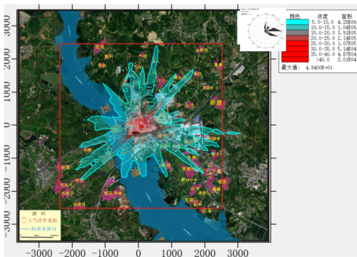
图 5.2-21 正常工况下氨小时均值贡献值预测图 (单位: \mu\text{g}/\text{m}^3 )
