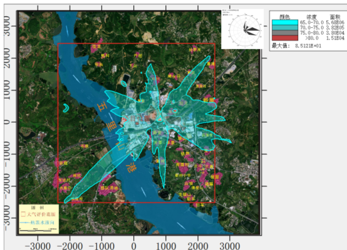
图 5.2-28 正常工况下 PM_{10} 日均值叠加背景值预测图 (单位: \mu g/m^3 )
