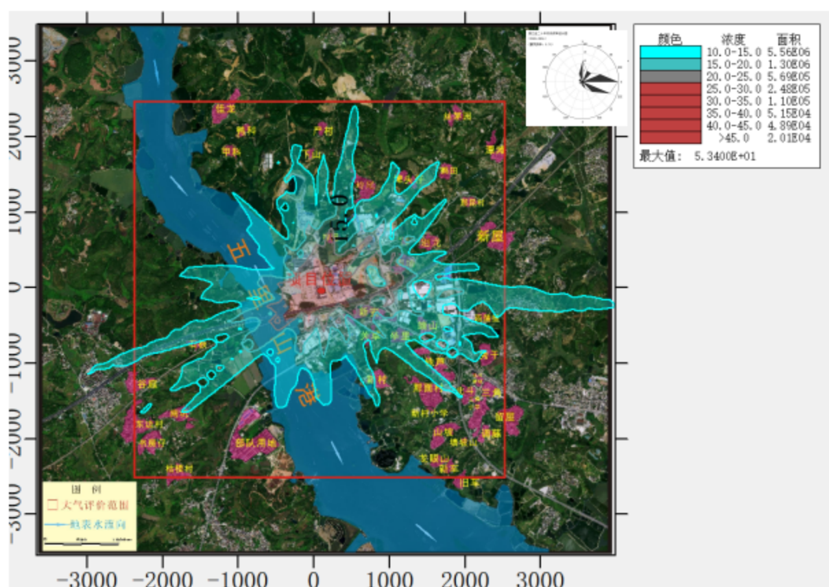
图 5.2-31 正常工况下氨小时均值叠加背景值预测图 (单位: \mu\text{g}/\text{m}^3 )
