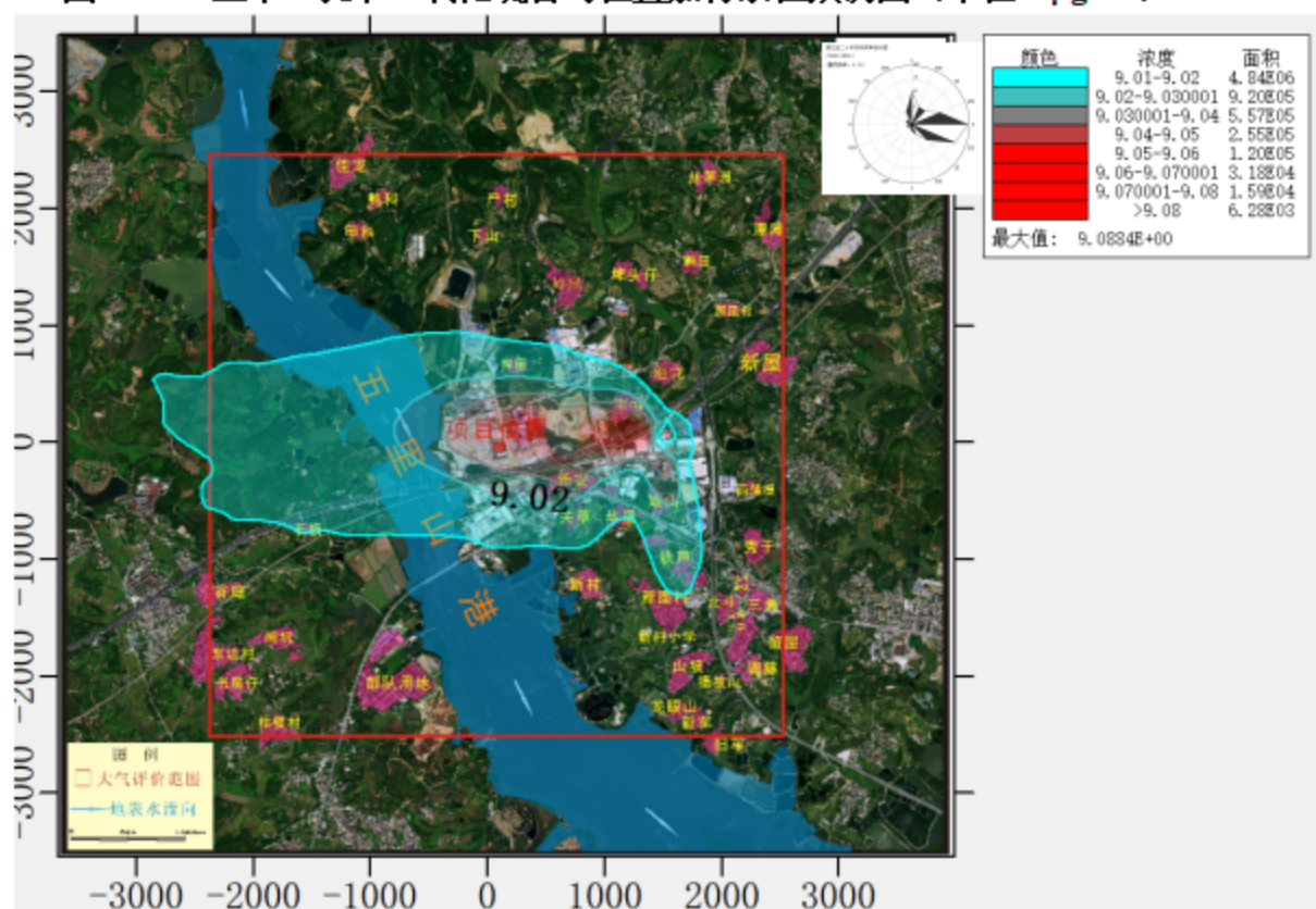
图 5.2-23 正常工况下二氧化硫年均值叠加背景值预测图 (单位: \mu\text{g}/\text{m}^3 )
