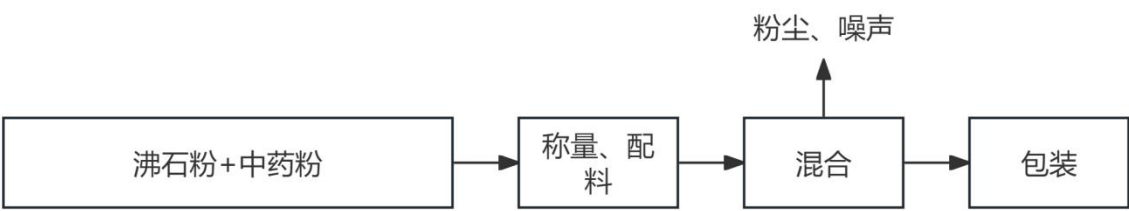
图 3.1-6 底改产品工艺流程图
