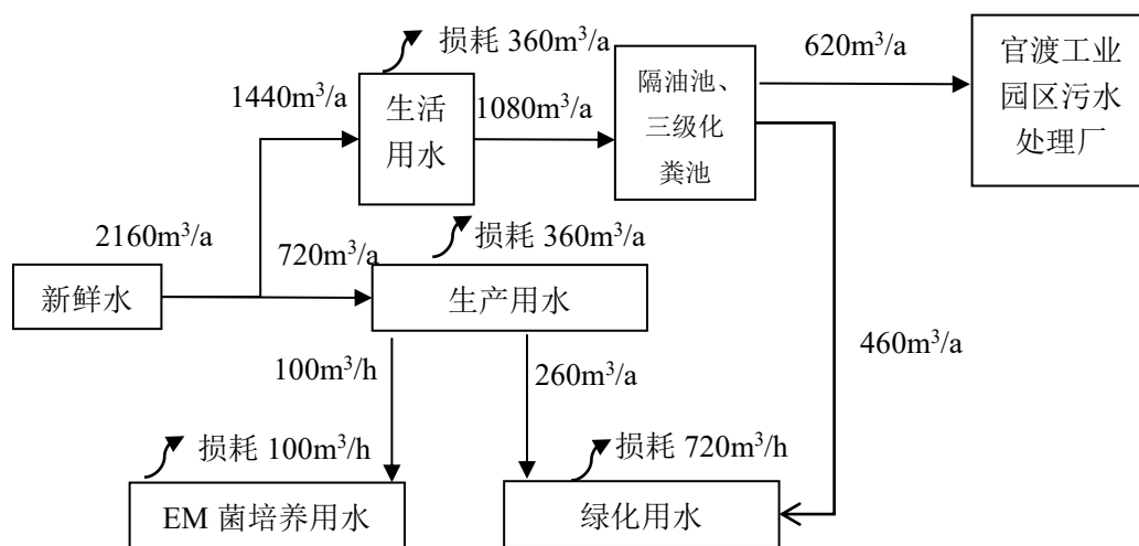
图 3.1-2 原有项目水平衡图 (m³/a)
