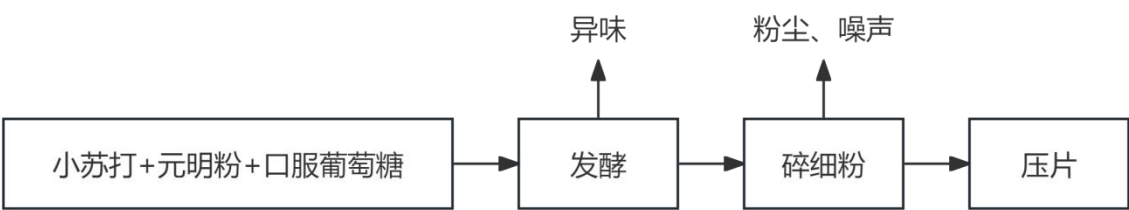
图 3.1-7 水质改良产品片剂工艺流程图
