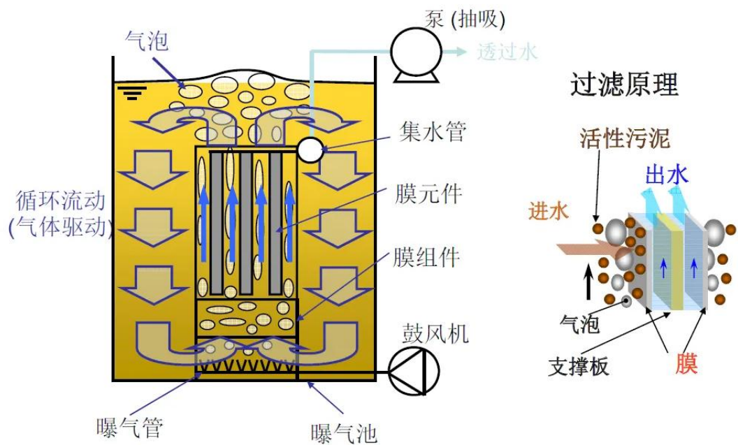
图 6.1-2 MBR 工艺原理示意图
